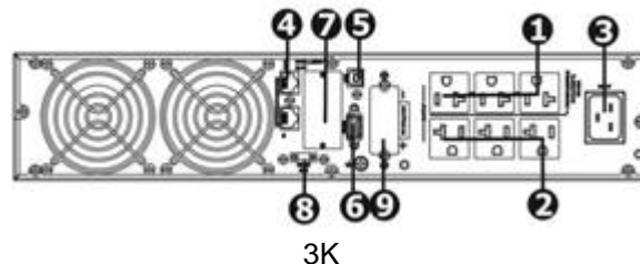
Vista do painel traseiro
