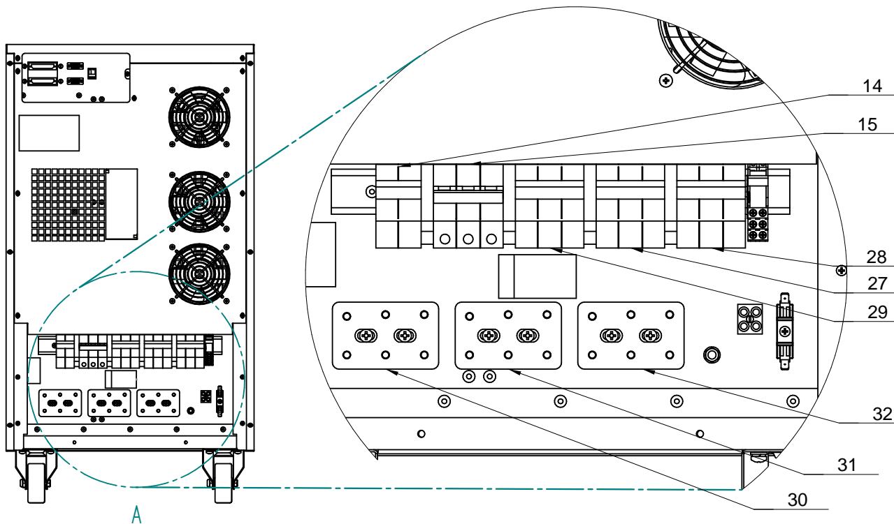
Detalhe Bornes
